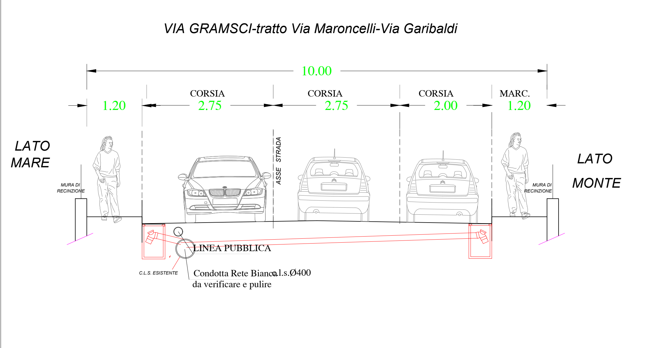
Sezioni tipo scala 1:50
